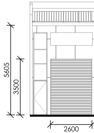
ELEVATION
